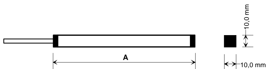
Fig. 2 Dimensioni - Dimensions
